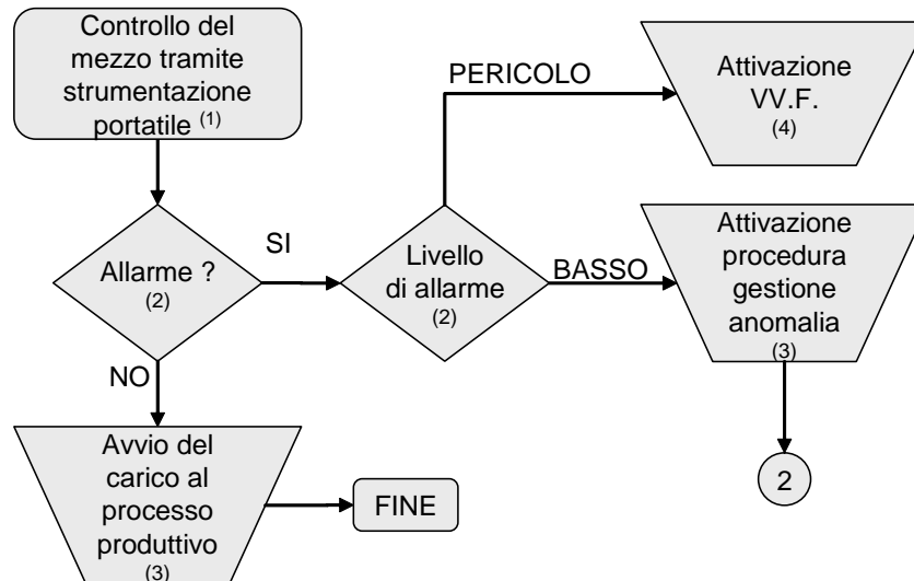
Figura 3.2 – Schema del flusso delle operazioni previste nella fase di sorveglianza radiometrica in ingresso all'azienda, effettuato per mezzo di strumentazione portatile
